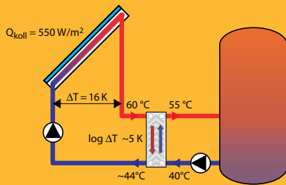
Tároló fűtés normál (high flow) térfogatárammal
