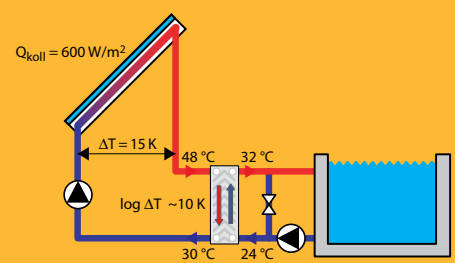
Medence fűtés normál (high flow) térfogatárammal
