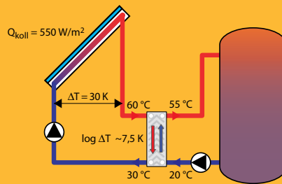
Tároló fűtés alacsony (low flow) térfogatárammal
